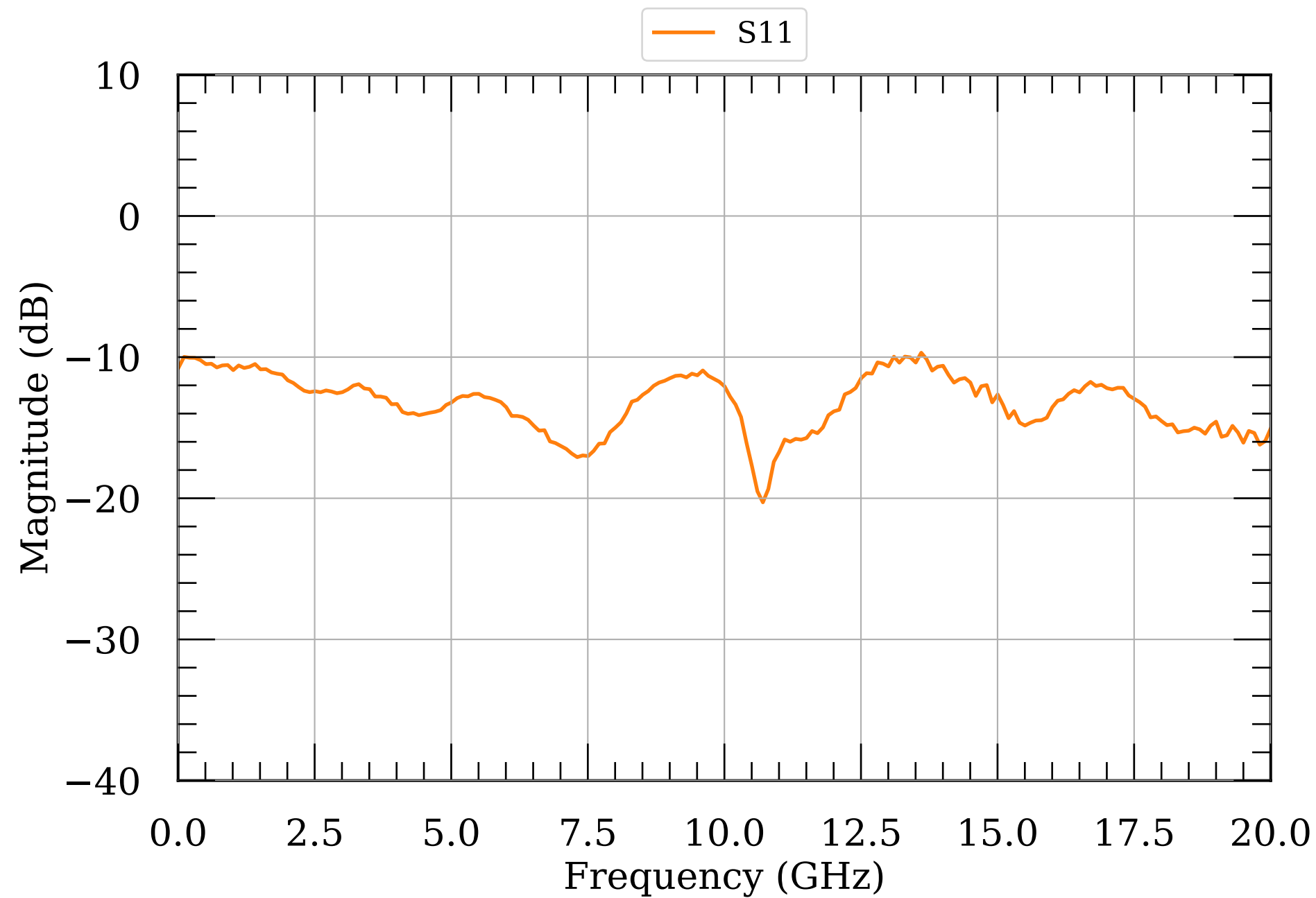
LNA S-params module088
